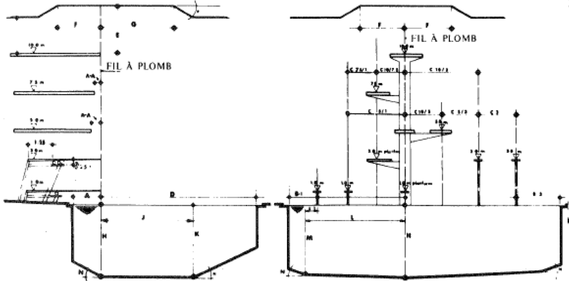
COUPE LONGITUDINALE
