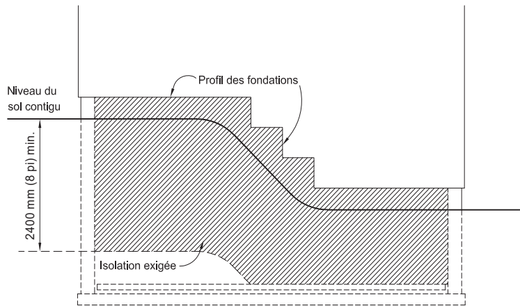
Figure A-3.2.3.1. 3) Isolation des murs en contact avec le sol ».
